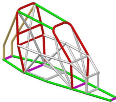
Figura 17 - Desenho 279B-1
