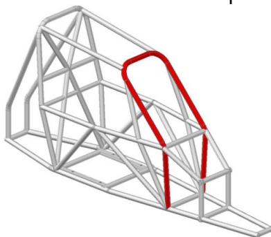
Figura 11 - Desenho 279B-4
