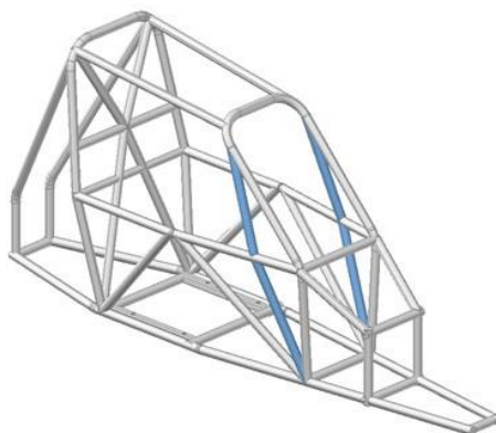
Figura 23 - Desenho 279B-11
