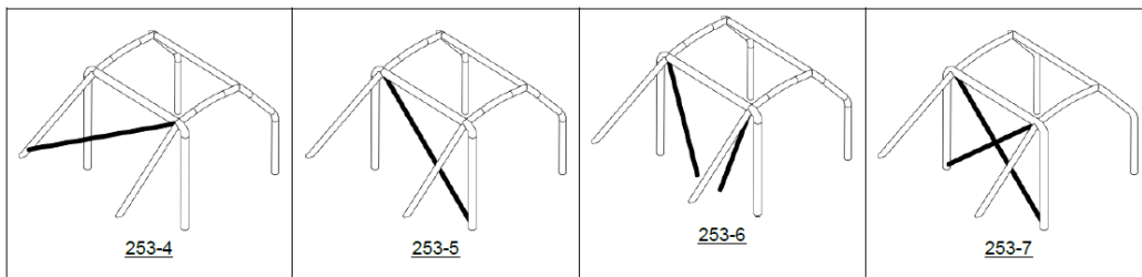
Figura 26 - Tipos de diagonais aceites - Anexo J - 253-4/5/6/7
