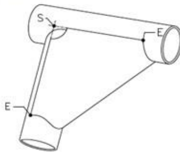
Figura 16 - Desenho 253-34
