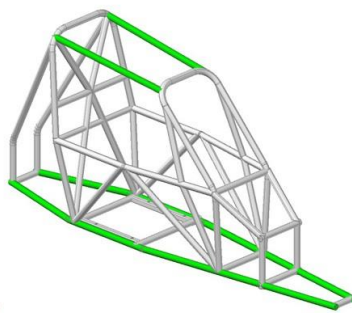
Figura 13 - Desenho 279B-6
