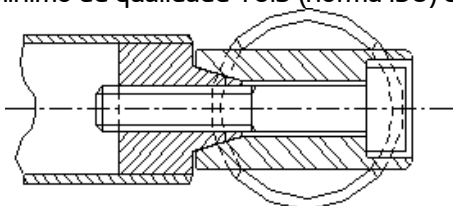
Figura 19 - Desenho 253-38
