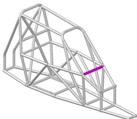
Figura 24 - Desenho 279B-12
