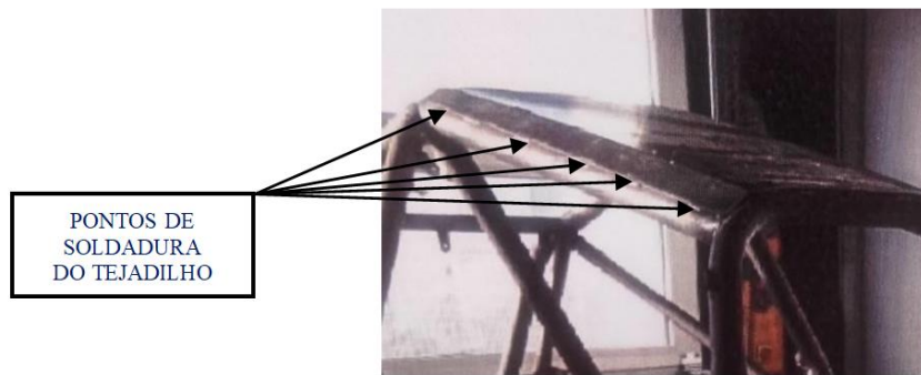
Figura 31 - Tejadilho
