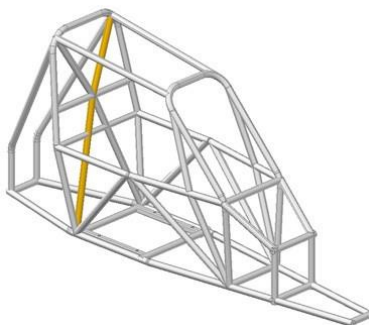
Figura 15 - Desenho 279B-8
