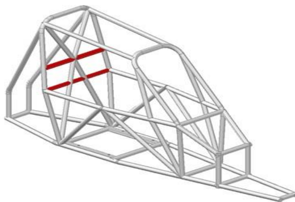
Figura 7 - Reforço transversal
