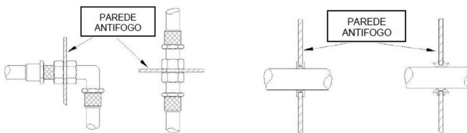
Figura 28 - Furações na parede antifogo - Anexo J - 253-59/60
