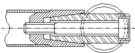
Figura 20 - Desenho 253-39
