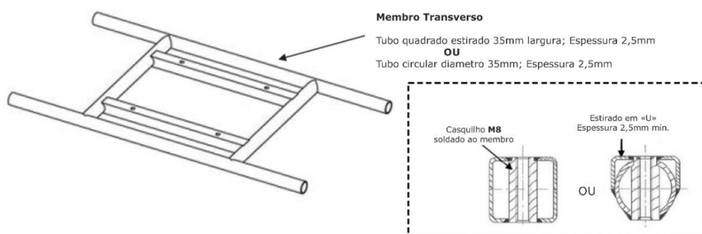
Figura 5 - Construção "D"
