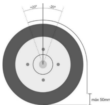
Figura 9 - Esquema de montagem dos guarda-lamas
