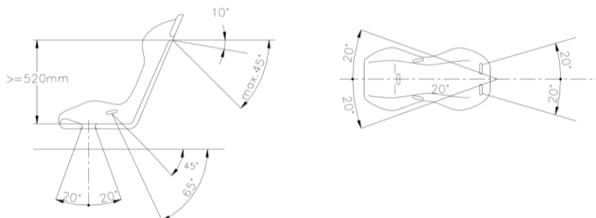
Figura 6 - Anexo J - 253-61
