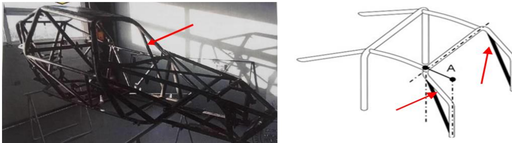
Figura 32 - Habitáculo / Reforço do montante do para-brisas
